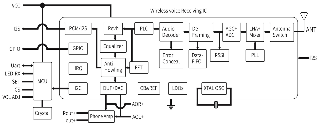
SA316-RX 方框图
