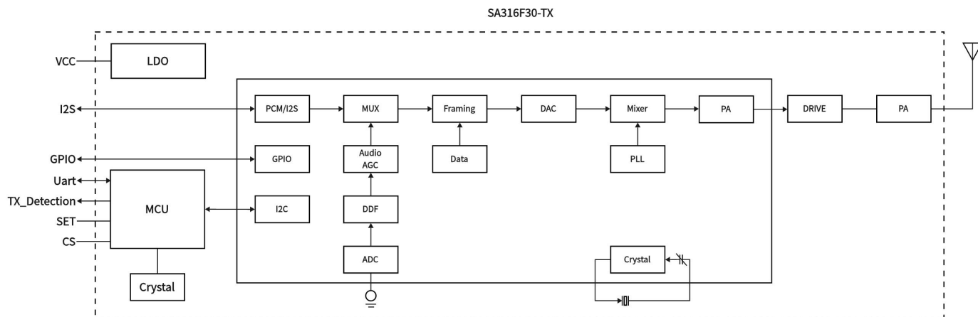
SA316S-TX 方框图
